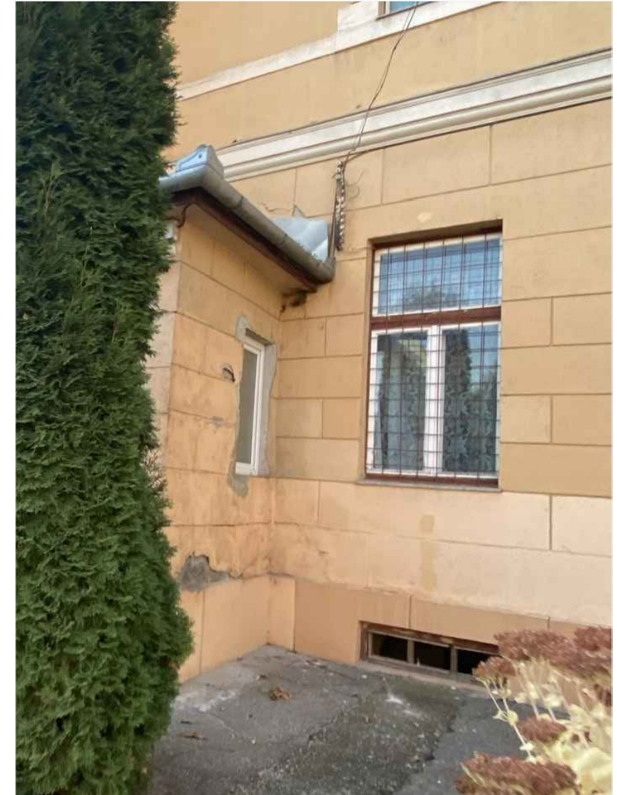
Tencuiala umflata/ desprinsa din cauza umiditatii de capilaritate si infiltratii. Lacune - diferente de culoare a tencuielii pe aceeaasi fatada.
